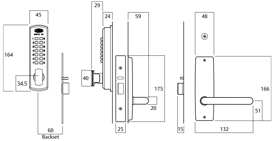
Backset
